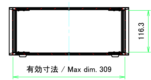
A-A ( 1 : 6 )
